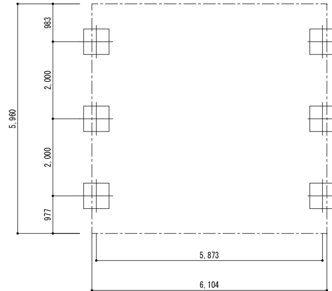
■ 基礎配置図
